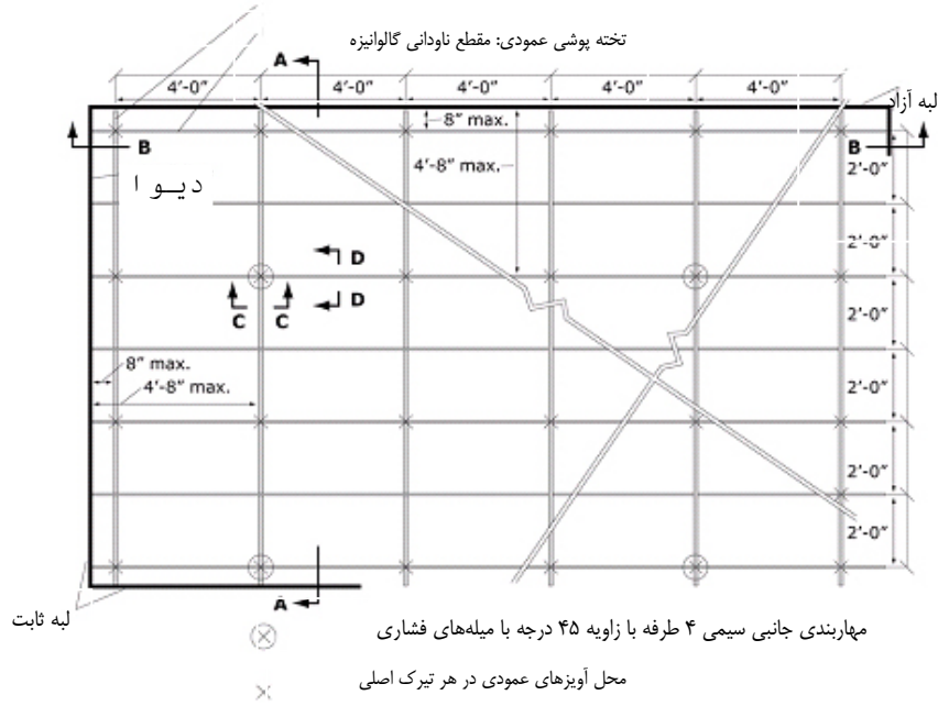
شکل پ-۳۳-۶- پلان مهربندی عرضی برای شبکه سقف سنگین معلق (جزئیات مقاطع نر شکل پ-۶-۲۹ ارائه شده است)
